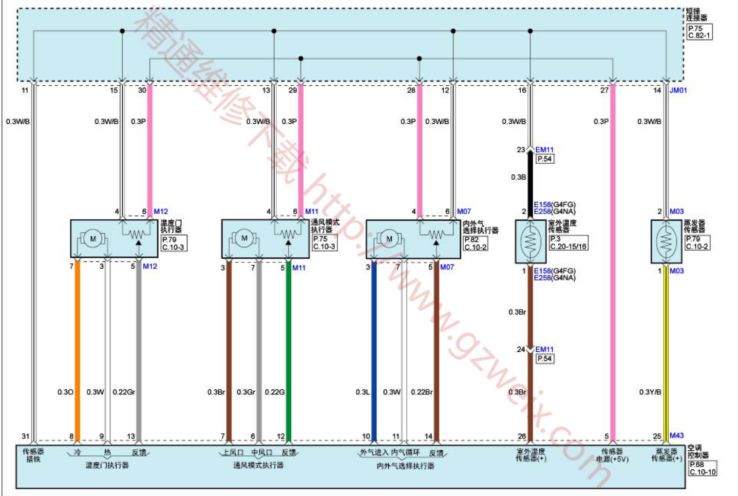
空调控制系统(手动)(2)
